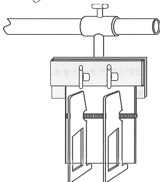
図 7 中板競技材の固定具と邪魔板の取り付け状況
