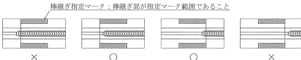
b) 初層棒継ぎ指定位置 30mm でアークスタートを行う場合
