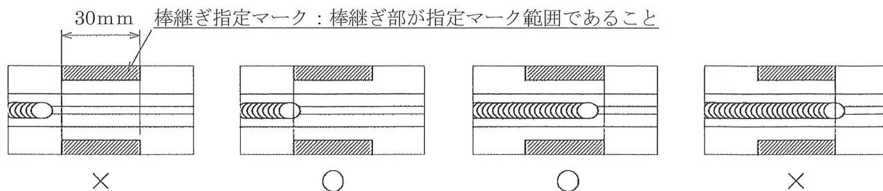
a) 初層棒継ぎ指定位置 30mm でアークを切る場合
