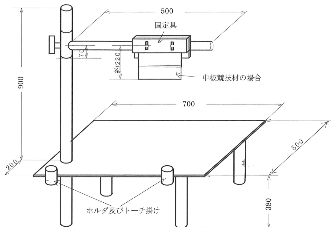
図 8 溶接作業台 全体図
