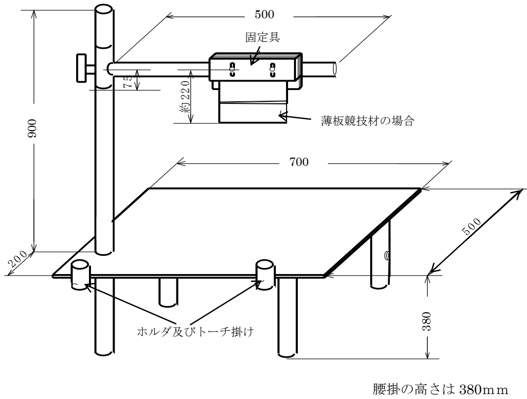
図8 溶接作業台 全体図
