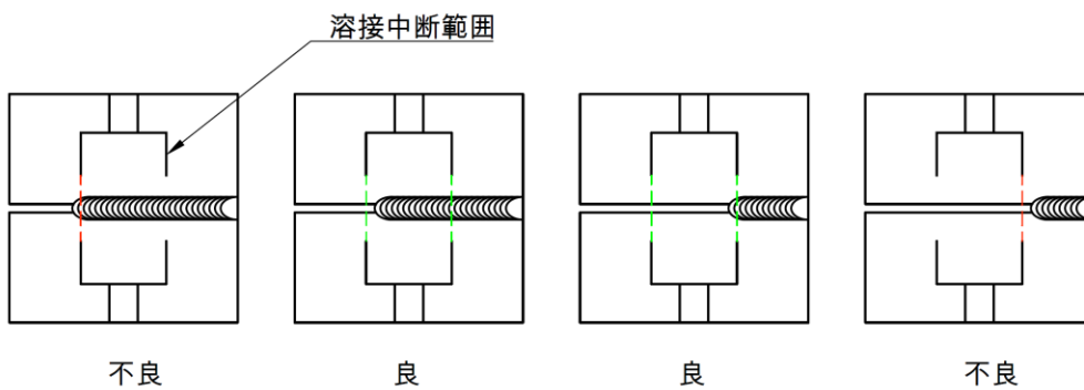
b) 溶接中断範囲でアークスタートを行う場合
